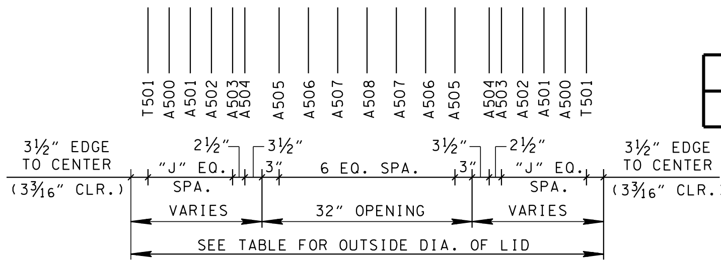
LID REINFORCING
